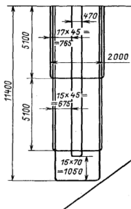
Рис. Размеры секции ширмового пароперегревателя
