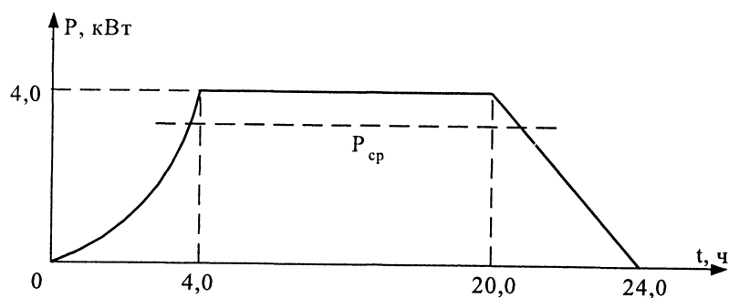
Рис. 4.23. Суточный график нагрузки
