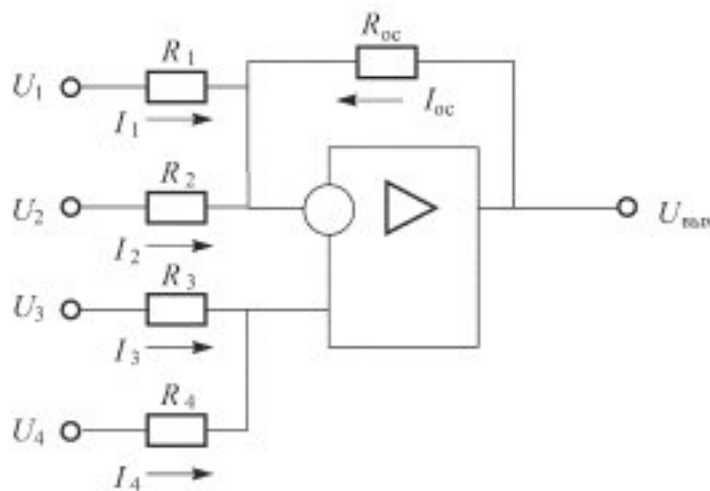
Рисунок 1. Схема суммирования
