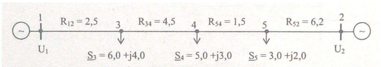
Рис. 5.1. Исходная схема
