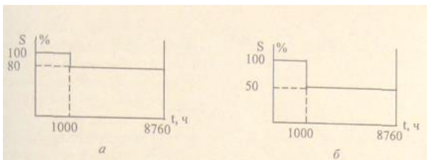
Рис. 6.1. Графики нагрузки по продолжительности
