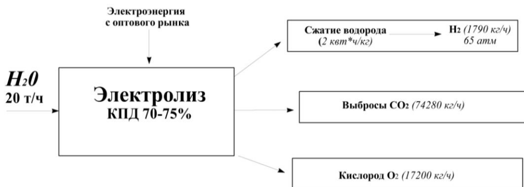
Рис. 1. Получение водорода методом электролиза с использованием электроэнергии с оптового рынка
