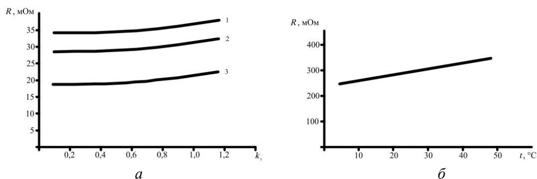
Рис. 2. a – зависимость сопротивления контактного соединения автоматического выключателя от температуры окружающей среды; б – сопротивления контактного соединения автоматических выключателей от срока эксплуатации:
