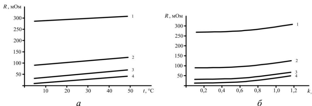
Рис. 1. a – зависимость сопротивления контактного соединения магнитных пускателей от температуры окружающей среды; б – сопротивления контактного соединения магнитных пускателей от коэффициента загрузки:
