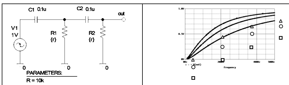
Рис. 2. Схема двойного RC -фильтра и его амплитудно-частотная характеристика ( R1 = R2 = 10 \text{ кОм} ( ), 15 \text{ кОм} ( ) и 20 \text{ кОм} ( )
