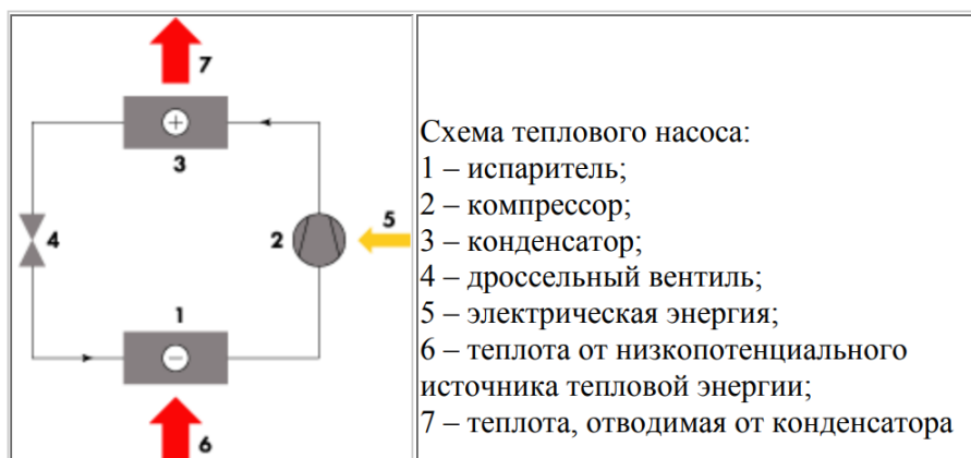
Тепловой насос
