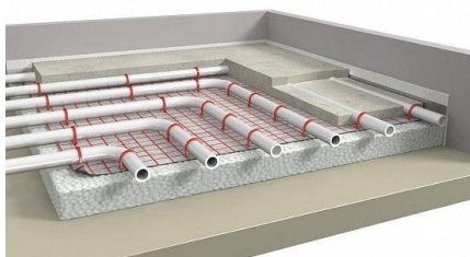
Рис. 2. Монтаж теплого пола
