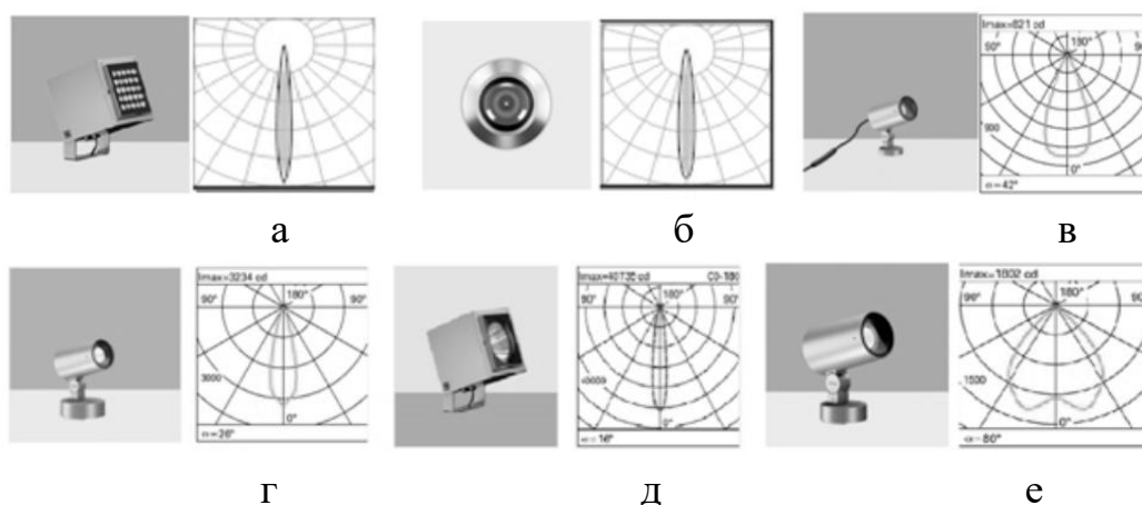
Рис. 2. Внешний вид и КСС используемых осветительных приборов а) iGuzzini BG 36_C418 ; б) iGuzzini EI01_B09C ; в) iGuzzini Q694_ B47B ; г) iGuzzini EH92_ B82B ; д) iGuzzini EP89_ C17BQ ; е) iGuzzini EI10_ B18C
