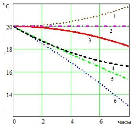
Зависимость температуры воздуха в помещении от времени
