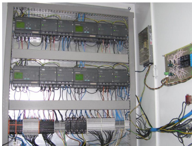
Рис .4. Шкаф системы автоматизированного контроля баллонов
